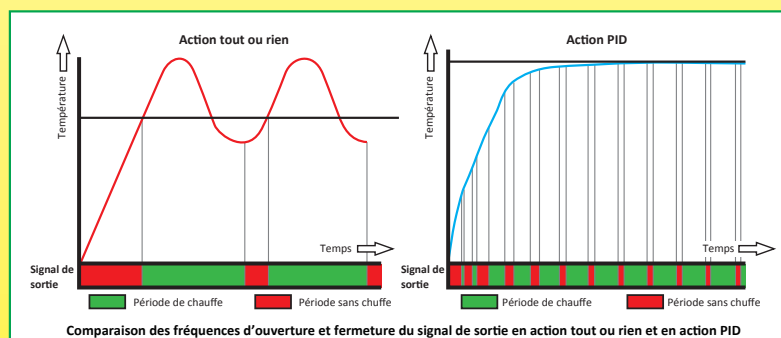
Comparaison des fréquences d'ouverture et fermeture du signal de sortie en action tout ou rien et en action PID
